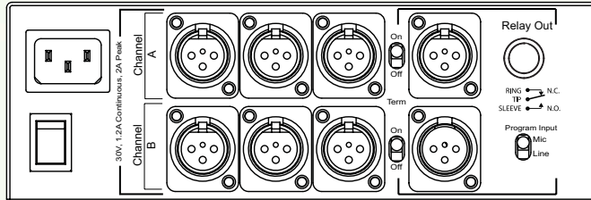
CS-702 Back Panel
