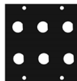
1/2BNC6 UCP Module, Six 1/2" BNC Punchouts
