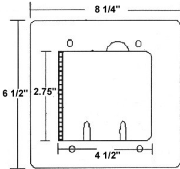
TOP VIEW LID
